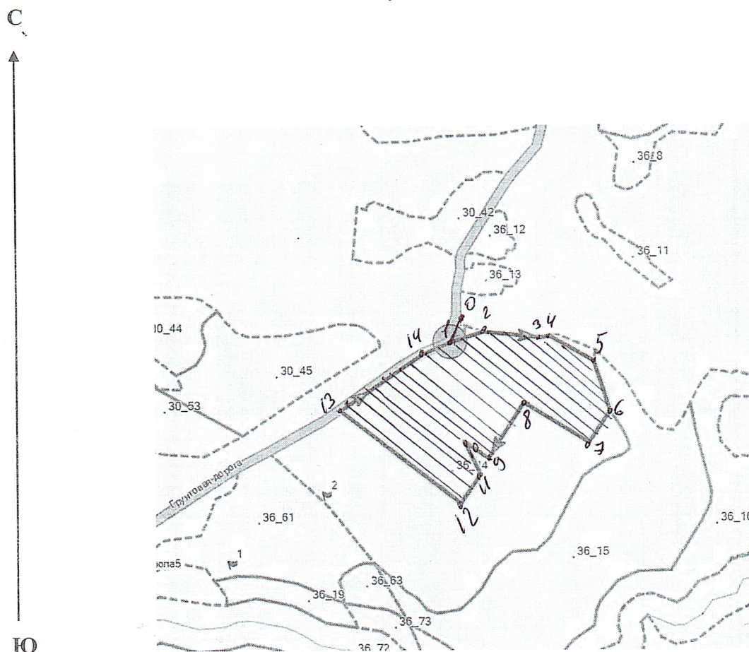
Общая схема участка и его привязки
