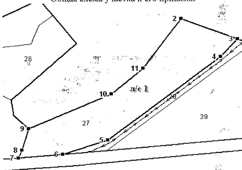
Общая схема участка и его привязки
