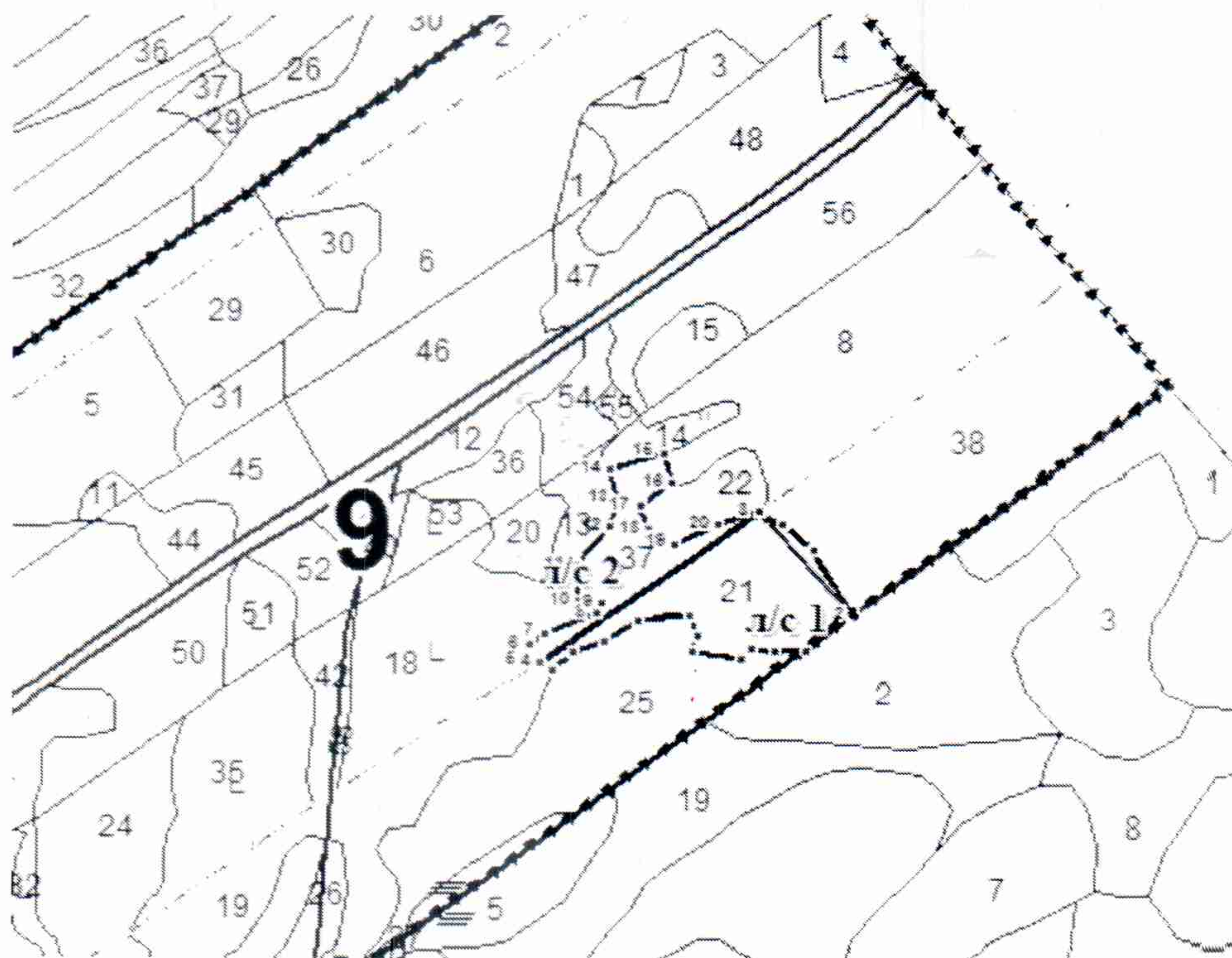
Общая схема участка и его привязки
